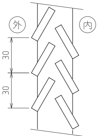
スレート部 詳細(S=1/2) 鉛戸式複葉型
